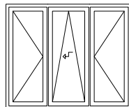
3-teiliges Element mit Schiebeflügel und zwei Drehflügeln
