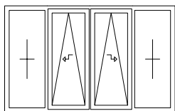
4-teiliges Element mit zwei Schiebeflügel und zwei Festverglasungen
