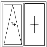
2-teiliges Element mit Schiebeflügel und Festverglasung
